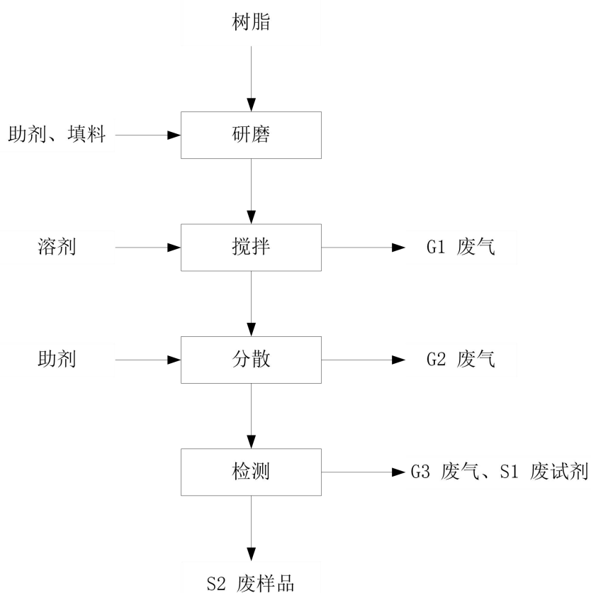
图 2-2 建设项目工艺流程图
